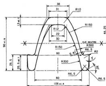
Perfil THN – 16,5
